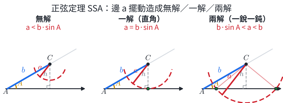
圖 1-4：SSA 模糊情況。固定角 A 與邊 b ，以 C 為圓心、半徑 a 畫弧（紅），弧與底邊的交點（綠）即三角形解。 a < b \sin A （短於高 h ）構不到底邊故無解； a = b \sin A 恰碰底邊一點（直角三角形）為一解； b \sin A < a < b 弧穿過底邊兩點為兩解。
